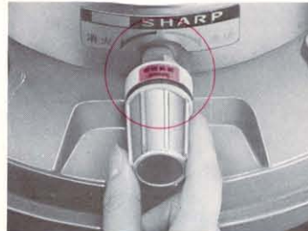
完全燃焼範囲に芯調節ツマミ表示線を合わせる 《燃焼表示ダイヤル》(HSA-83、HSA-84)
