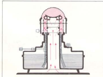
ニオイ、ススなし…バーナーも特別設計 《完全燃焼バーナー》
